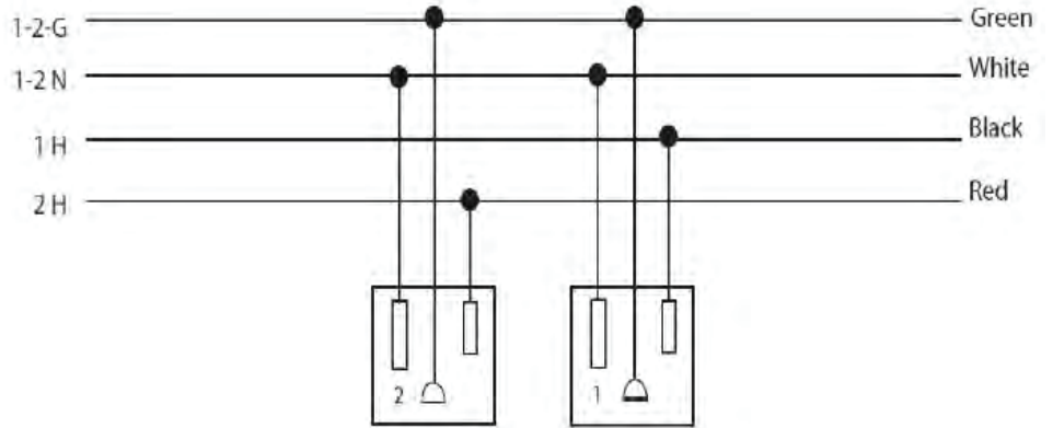
Wiring schematic
